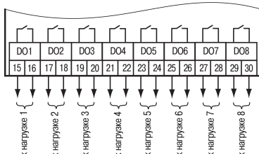
Рисунок 10 – Схема подключения нагрузки к ВЭ типа «Р»
