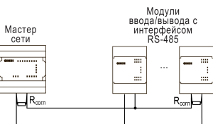
Рисунок 12 – Типовая схема подключения для ПР100 в режиме Master
