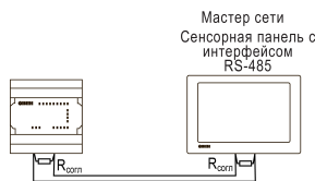
Рисунок 11 – Типовая схема подключения для ПР100 в режиме Slave
